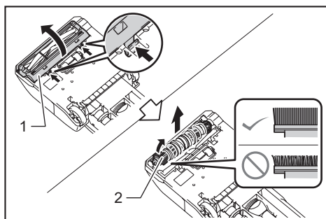
► 1. Plaque inférieure 2. Rouleau-brosse
