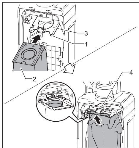
► 1. Fente 2. Sac filtre 3. Support 4. Loquet
