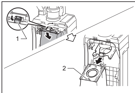
► 1. Loquet 2. Bande
