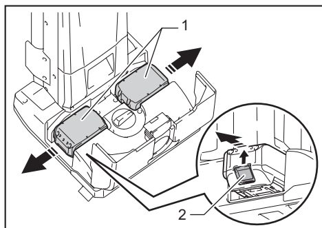
► 1. Batterie 2. Bouton
