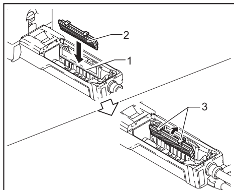
► 1. Rainure 2. Filtre HEPA 3. Crochet
